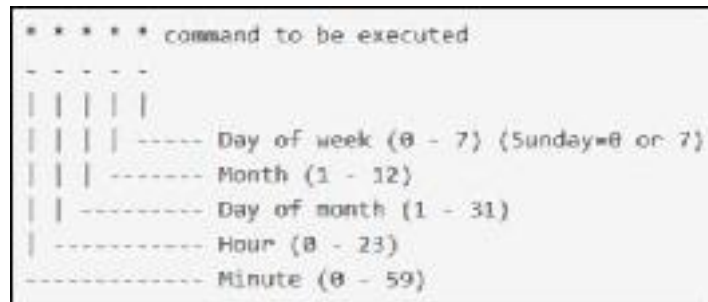
Gambar 2.5 Penjelasan Format Crontab
