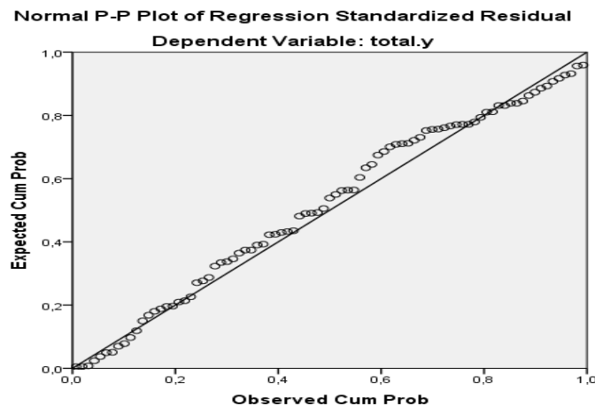
Gambar 1 Hasil Pengujian Normalitas
